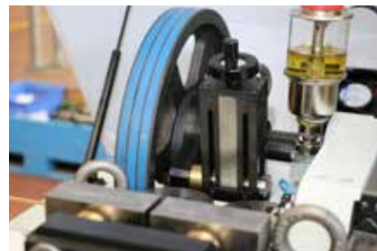
切削长度调整机构
